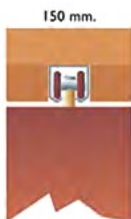
FIG. A Marco de 150 mm. con RIEL OCULTO sobre marco, y puerta totalmente enrasada.
