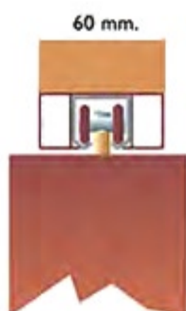
FIG. B Marco de 60 mm. RIEL ENFUNDADO
